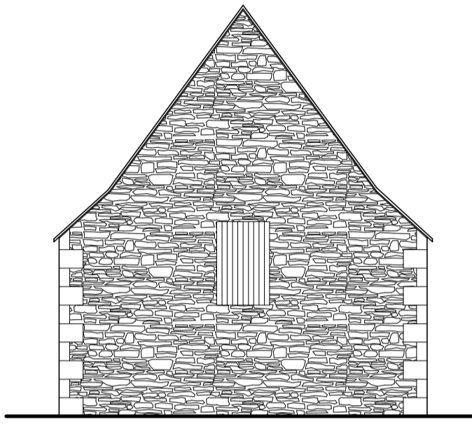
Existant Facade Ouest
