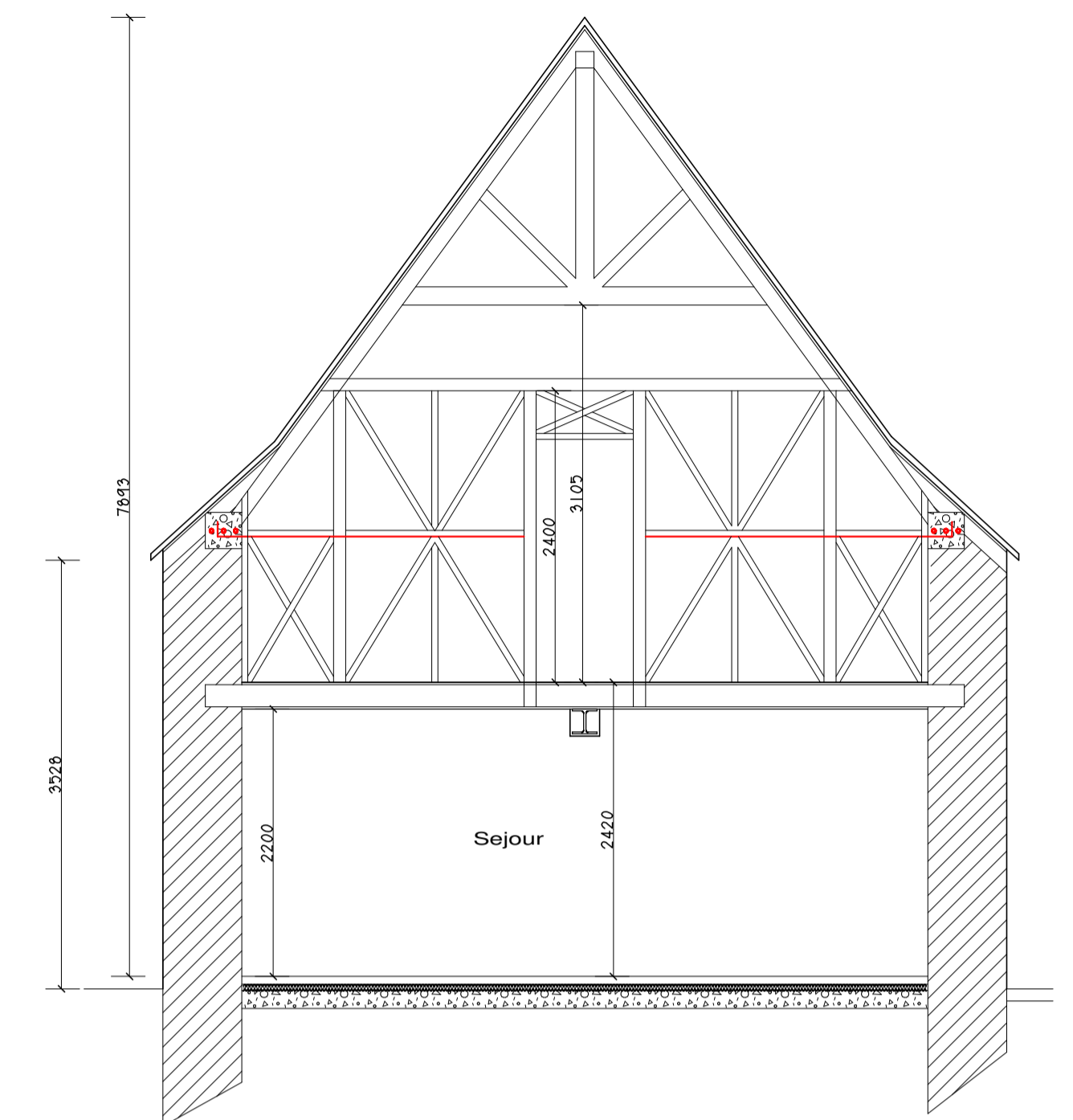
Coupe A-A (echelle 1:50)
